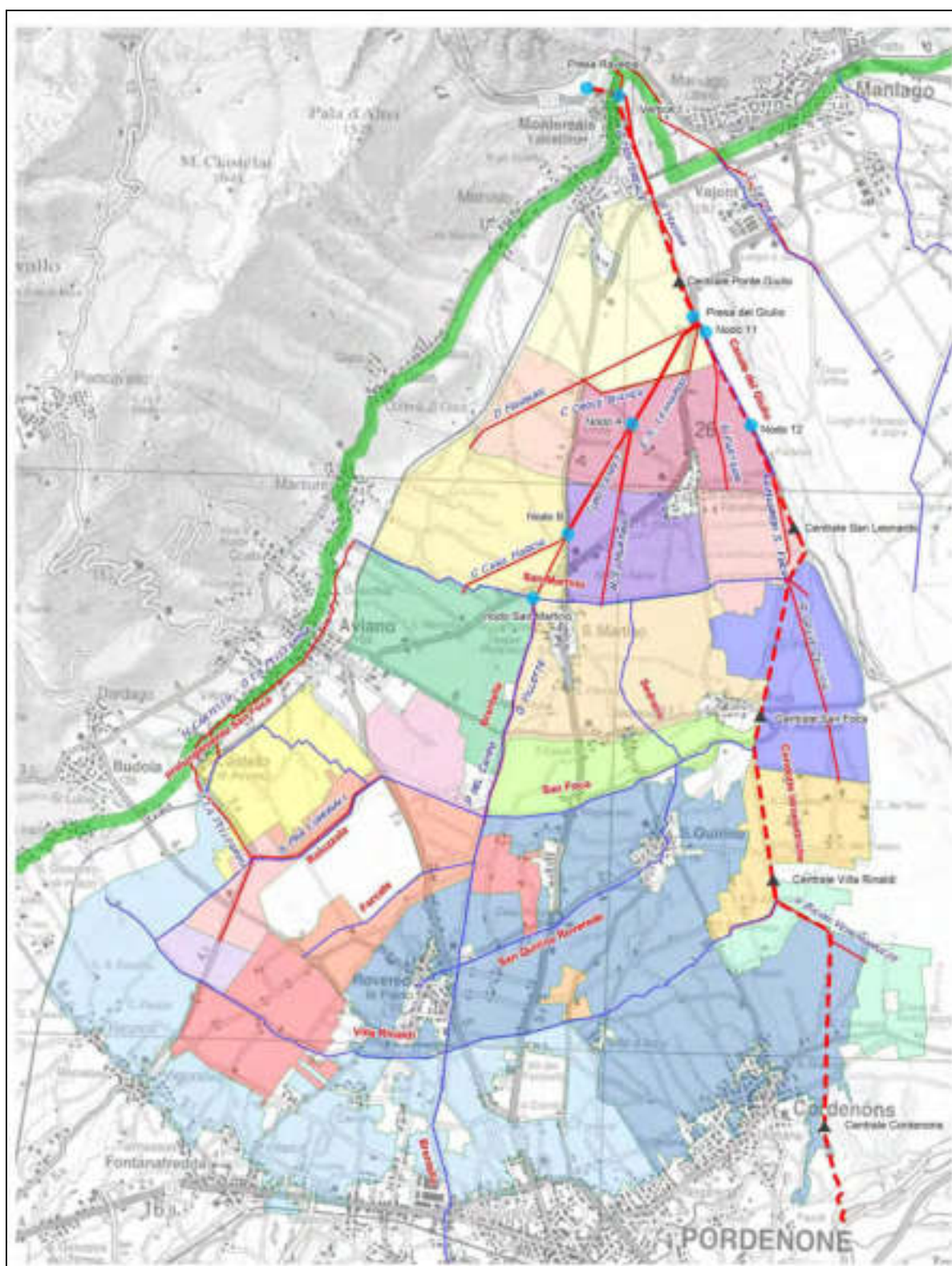
Figura 9 – In rosso le condotte principali della zona Cellina – in blu i canali
