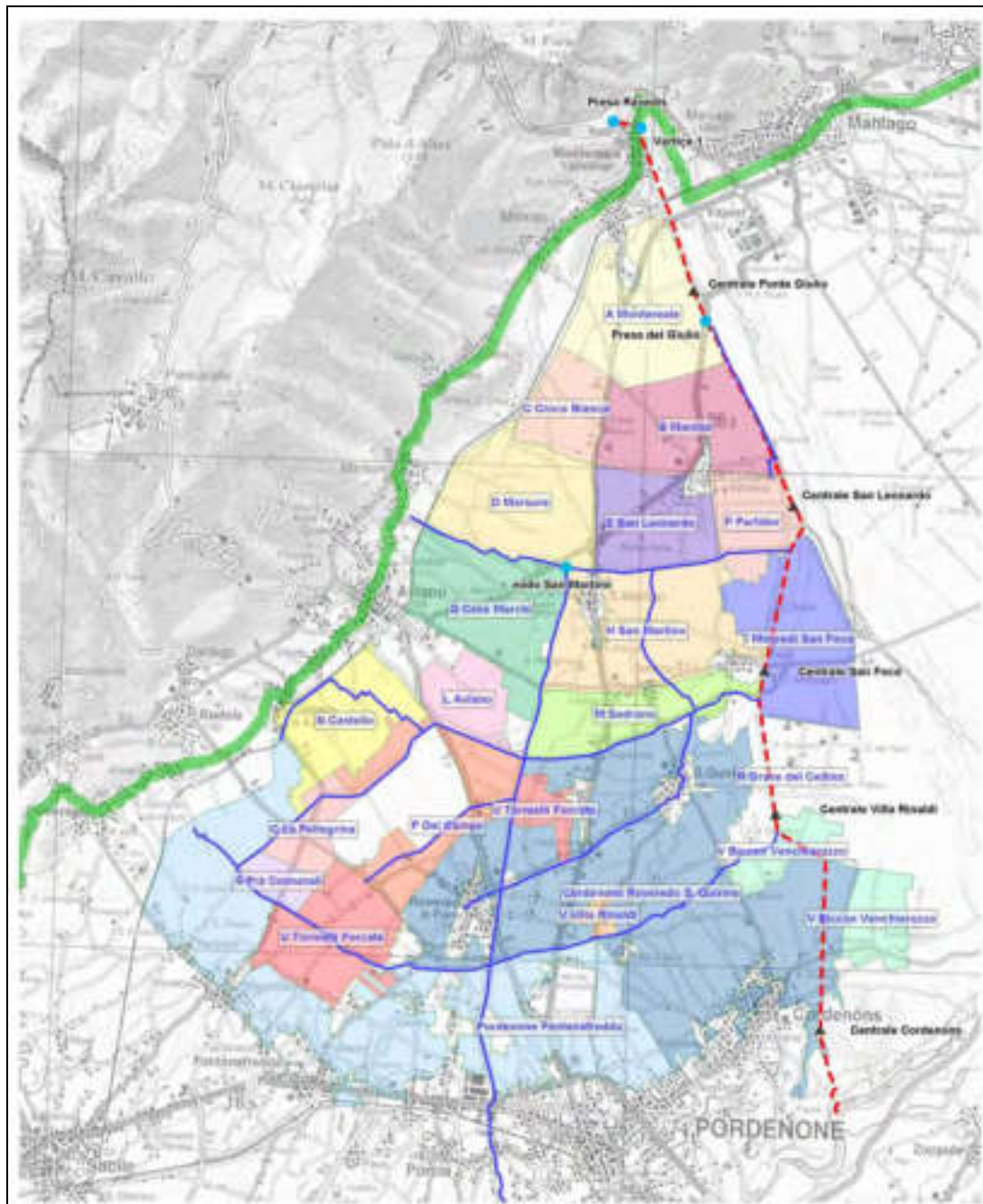
Figura 6 - Compartimenti irrigui della zona Cellina
