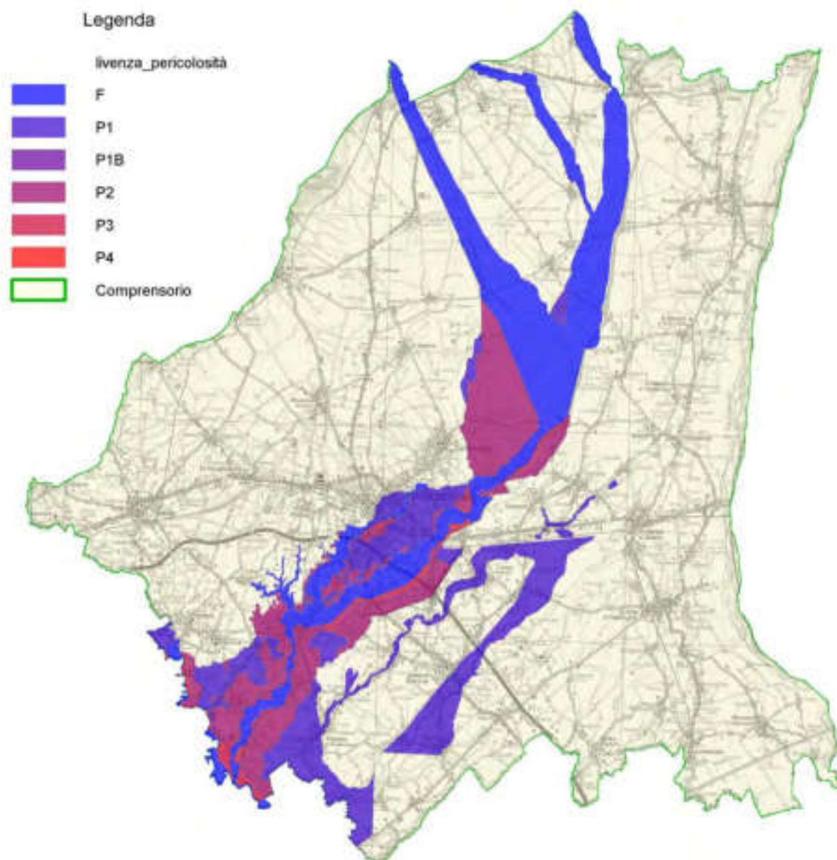
Figura 23 - Carta della pericolosità idraulica nel bacino del Livenza
